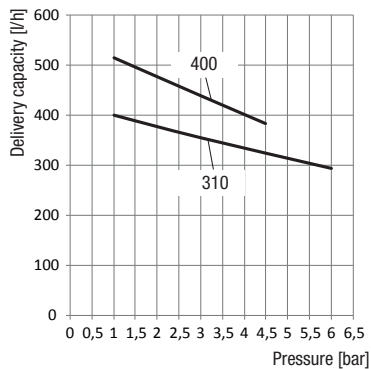
MEMDOS 310, 400
