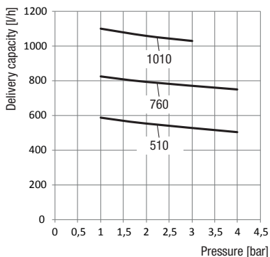
MEMDOS 510, 760, 1010
