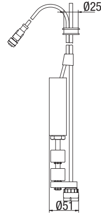
Fig. 3: Type SL-2
