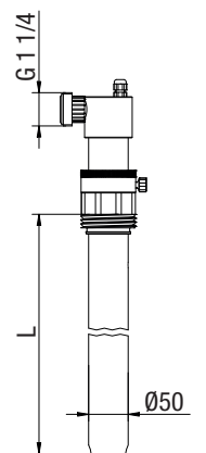
Fig. 12: Type SDL-2 DN15
